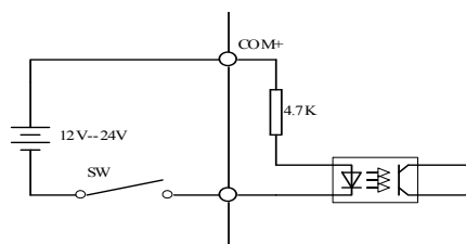
图 3.5.1 Type1 开关量输入接口
