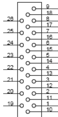
图 3.4b 接 CN2 的插头（DB26-3 针）管脚排列
