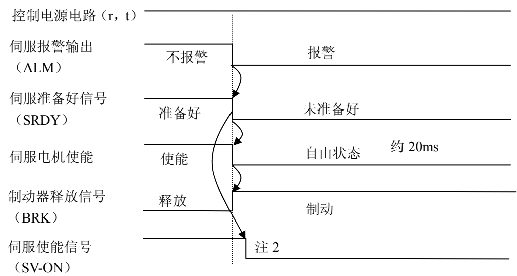
图 7.2.2b 报警时序图
