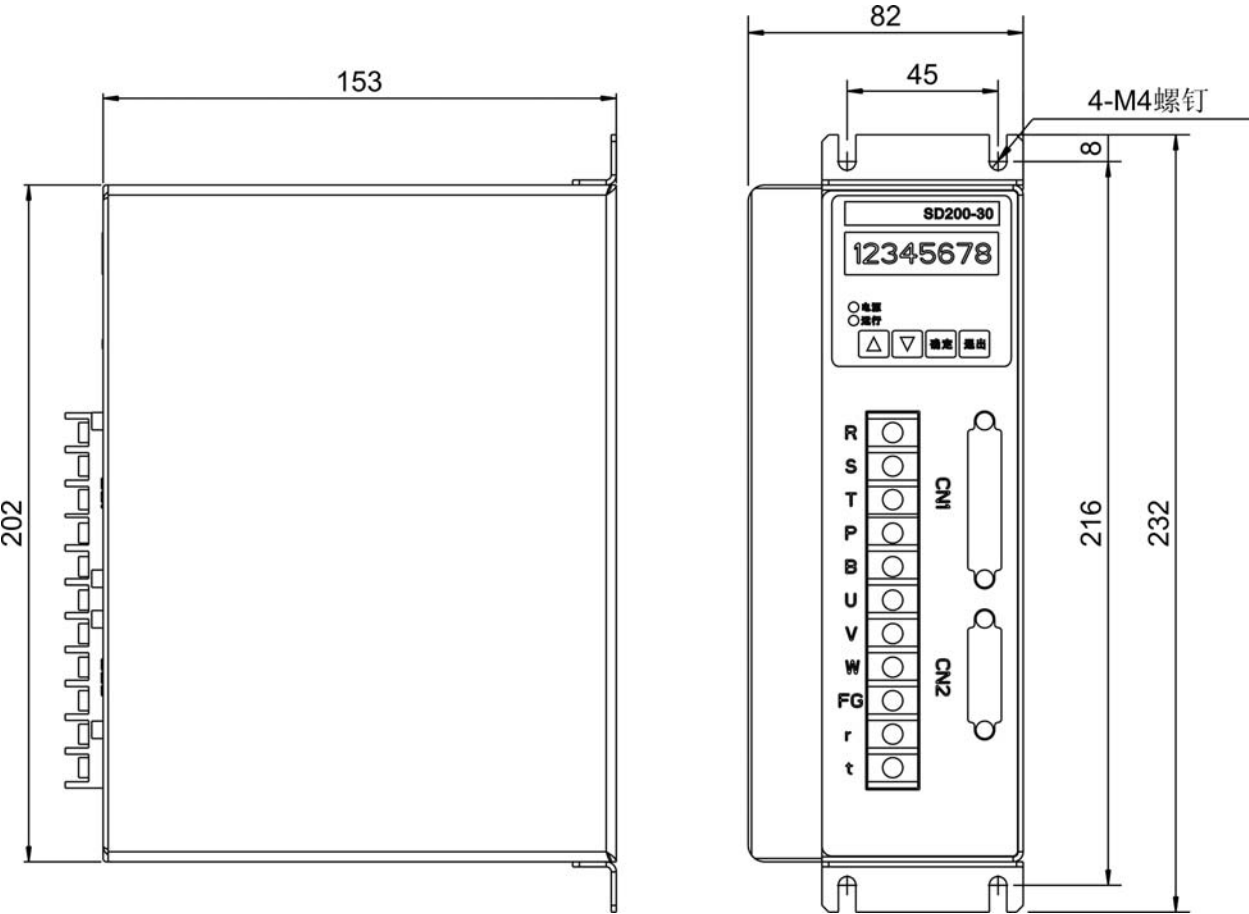
图 1-2 KND SD200-30 安装尺寸图
