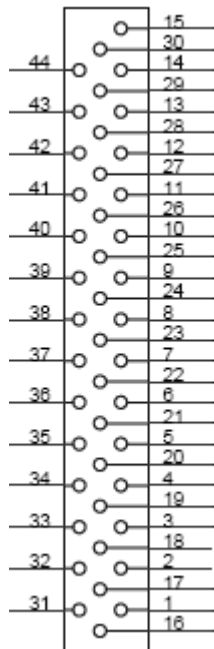
图 3.4a 接 CN1 的插头（DB44-3 针）管脚排列
