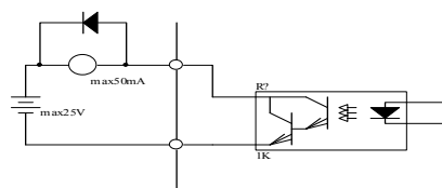
a.继电器连接
